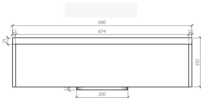
VISTA TRASEIRA
