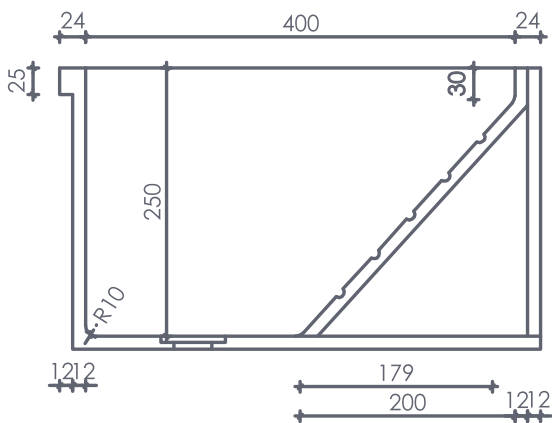
CORTE
