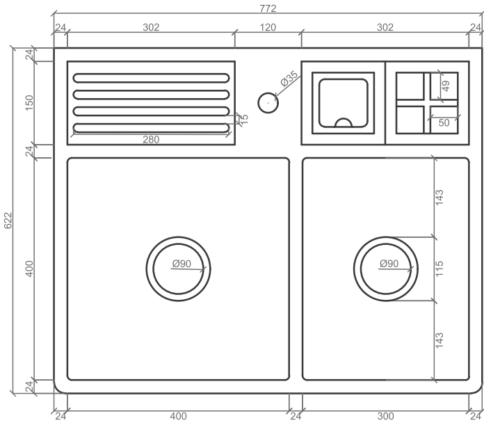
VISTA SUPERIOR
